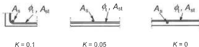
Figur 8.4 – Verdier av K for bjelker og plater
