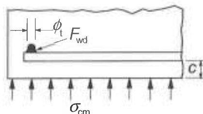
Figur 8.6 – Sveiste tverrgående stenger som forankringsenhet
