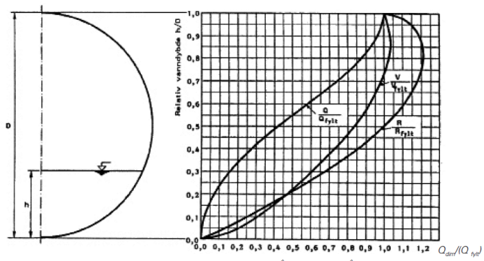
Figur 2. Delfyllingsgraden for avløpsrør /2/
